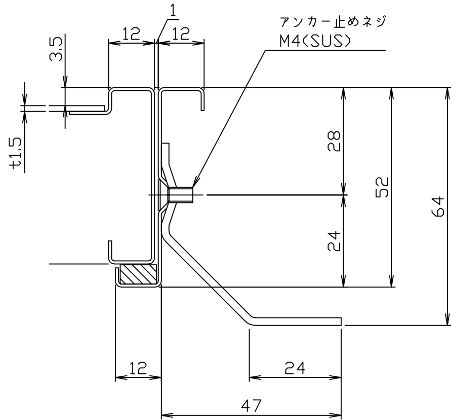
断面詳細
