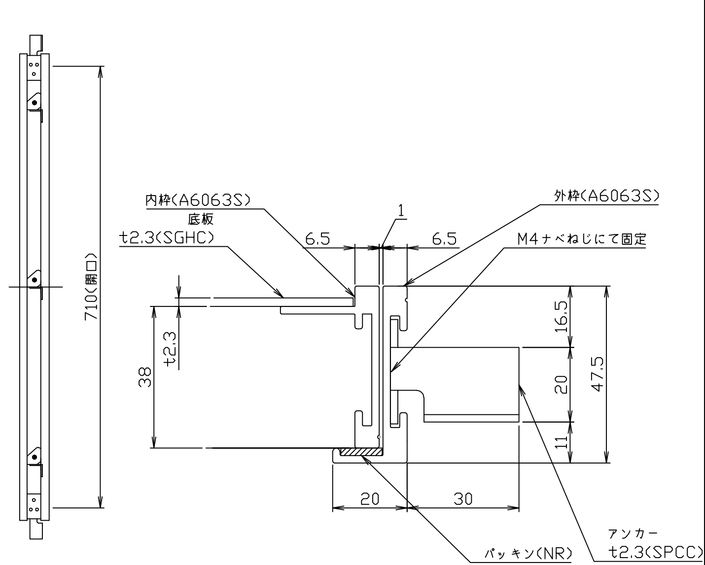
枠断面詳細
