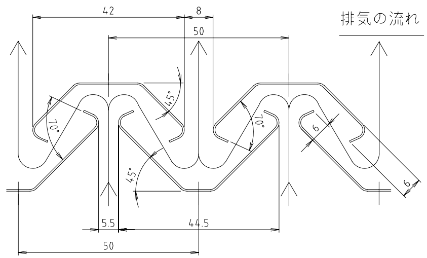
衝突板断面
