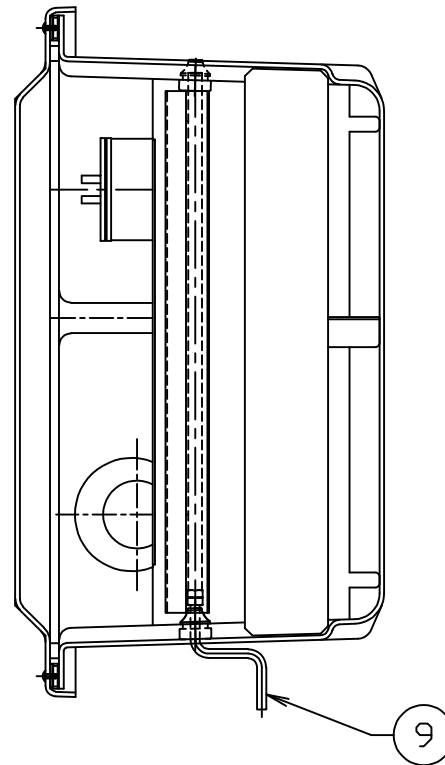
B-B'断面
