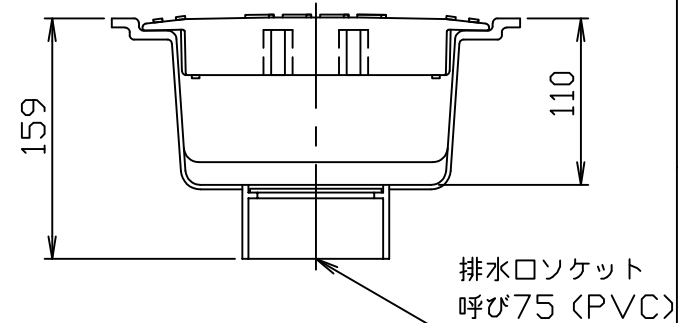
排水部断面詳細図
