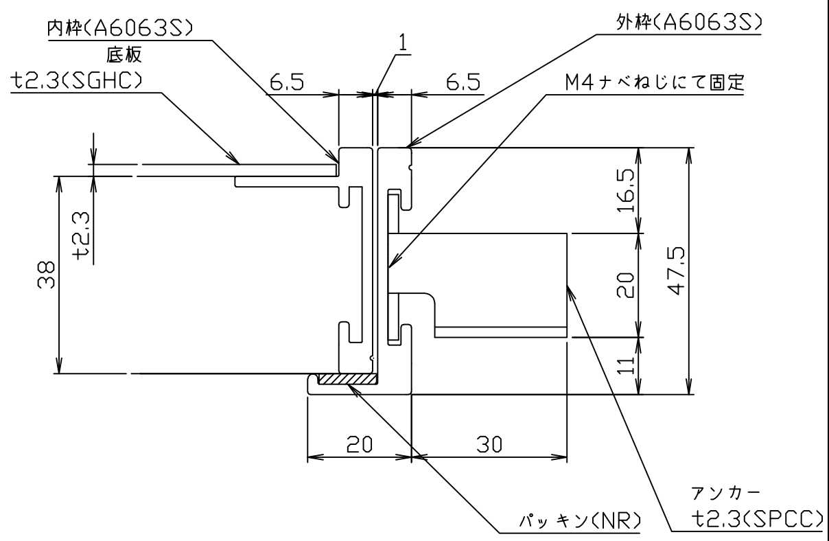
断面詳細
